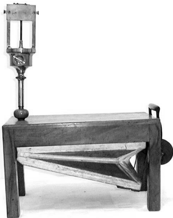
N° 147 – Sirena di Cognard de la Tour
