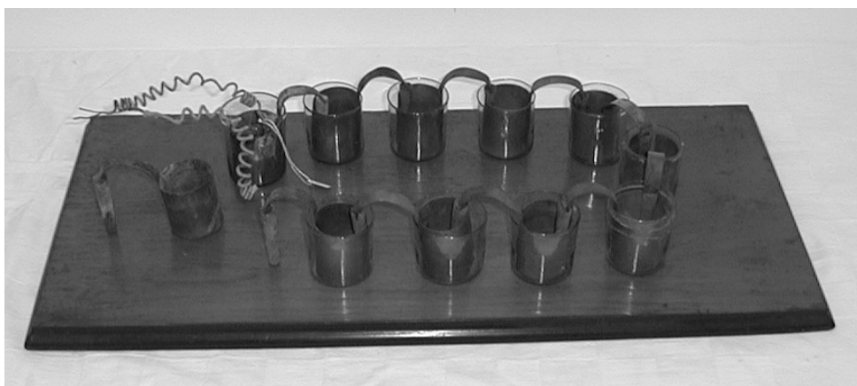
N° 275a – Pila a corona di tazze
