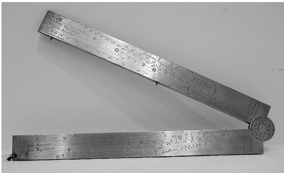
N° 13 – Compasso di proporzione di Lusverg
