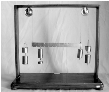
N° 24 – Apparecchio per le forze parallele
