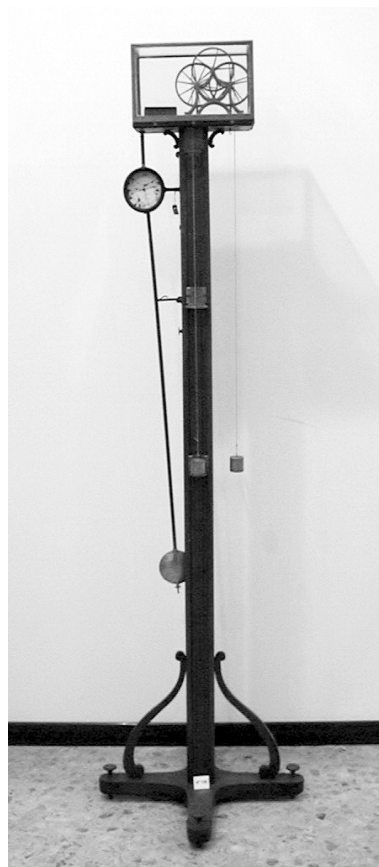
N° 126 – Macchina di Atwood
