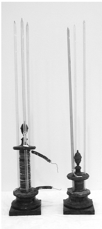
N° 272 – Vecchie pile a colonna
