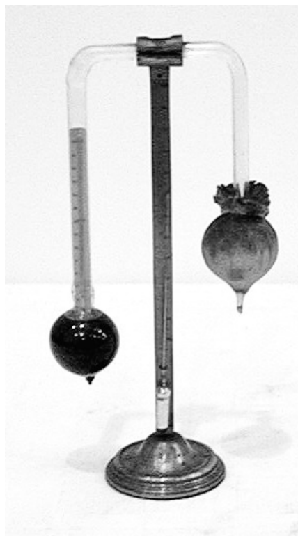
N° 81 – Igrometro di Daniell
