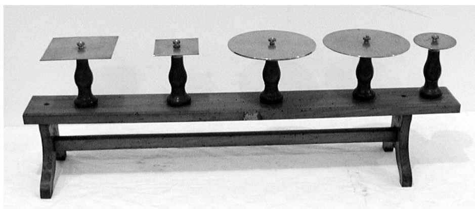
N° 163 – Apparecchio di Chladni
