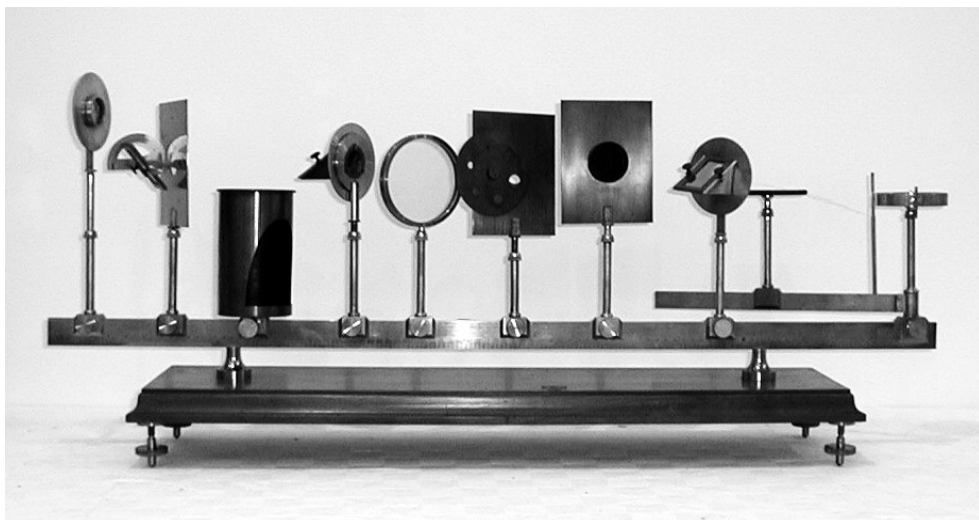
N° 469 – Apparato di Melloni completo
