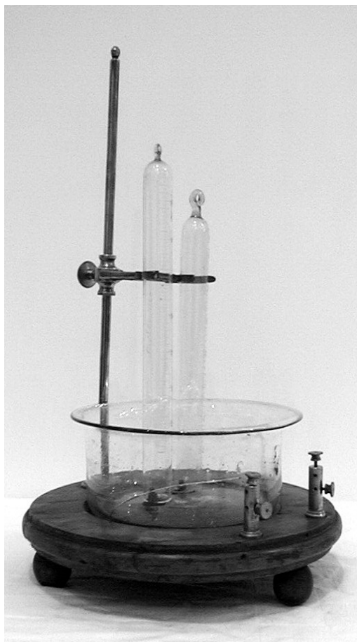
N° 563 – Voltmetro di Bertrand
