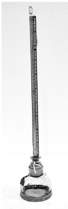
N° 42 - Endosmosometro
