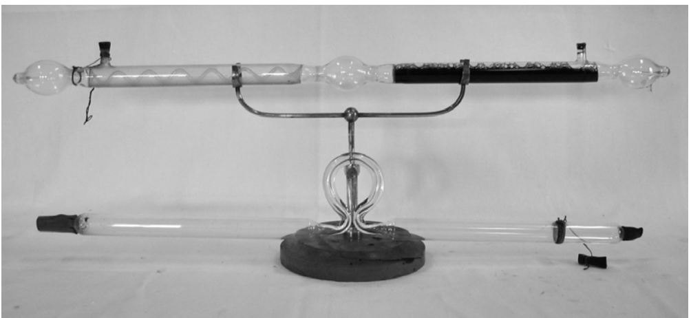
N° 330 – Tubi di Geissler
