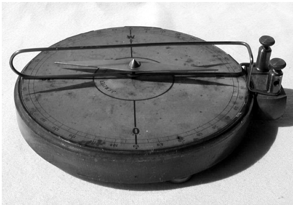
N° 298 – Apparecchio di Oersted
