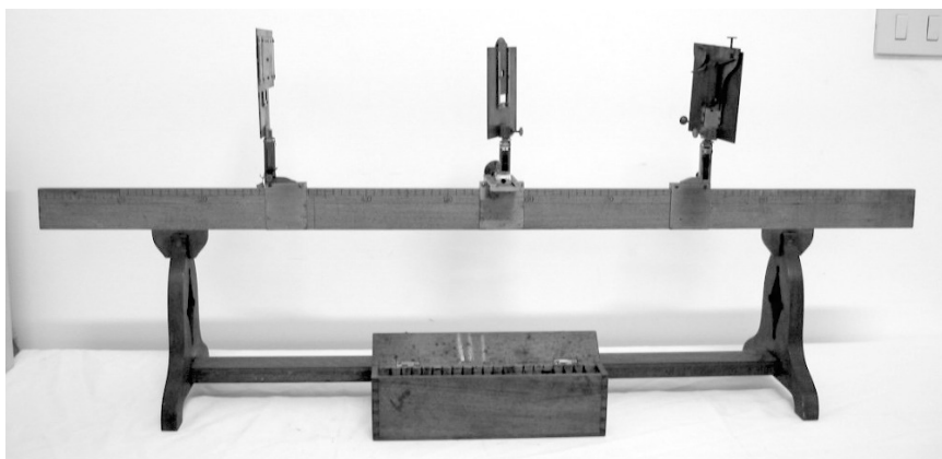
N° 211 – Banco di diffrazione col suo corredo
