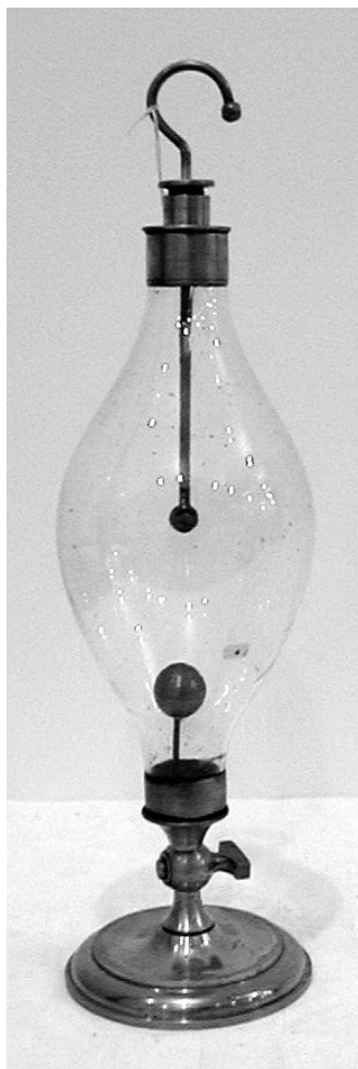
N° 248 – Ovo elettrico
