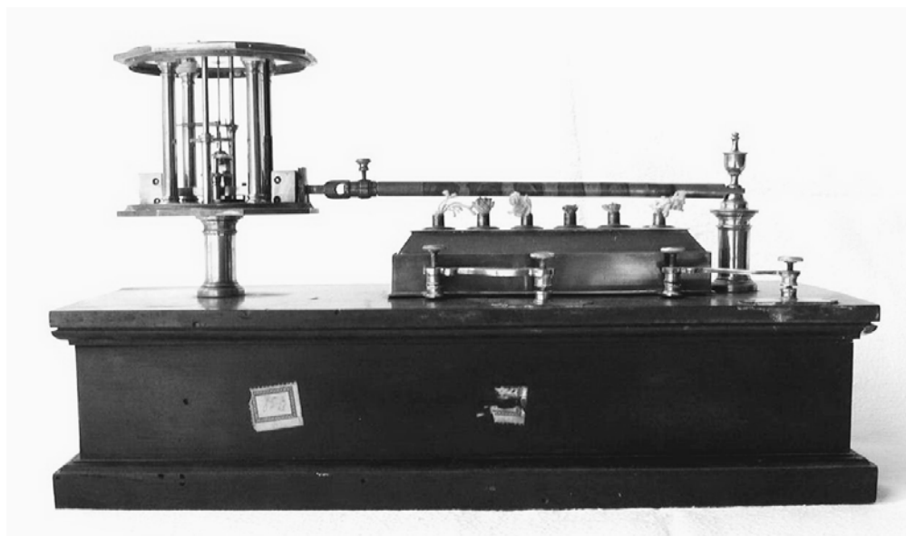
N° 85 – Pirometro a quadrante
