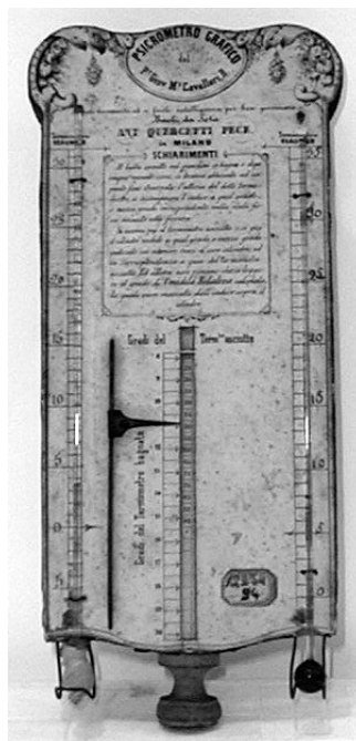
N° 94 – Psicrometro di Cavalieri
